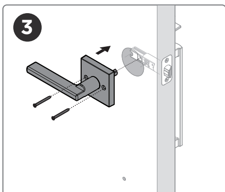
Secure interior lever with mounting screws Palanca interior segura con tornillos de montaje Levier intérieur sécurisé avec vis de fixation
