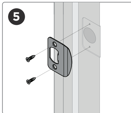
Install lever strike Instale la place de la manija Installer une gâche à levier
