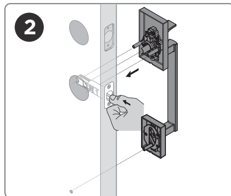
Install exterior grip on door Instalar el tirador exterior en la puerta Installer une poignée extérieure sur la porte
