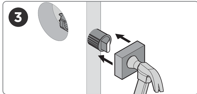
Slightly hammer latch into place using wood block Fije el pestillo golpeándolo ligeramente con un bloque de madera
