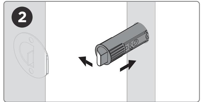
Install the latch with the slanted surface facing the strike Instale el pestillo con la superficie inclinada orientada hacia el cerrojo
