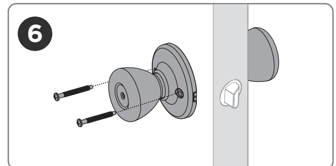
Install mounting screws Instale los tornillos de montaje
