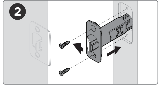
Install the latch with the slanted surface facing the strike Instale el pestillo con la superficie inclinada orientada hacia la placa Installez le loquet avec la surface inclinée forientée vers la gâche
