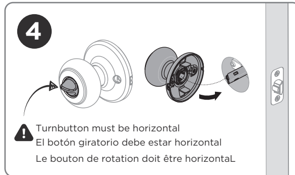
Install the interior Instale el interior Installer l'intérieur
