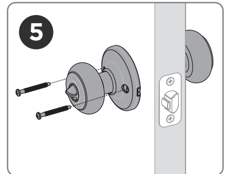
Install mounting screws Instale los tornillos de montaje Installez les vis de montage
