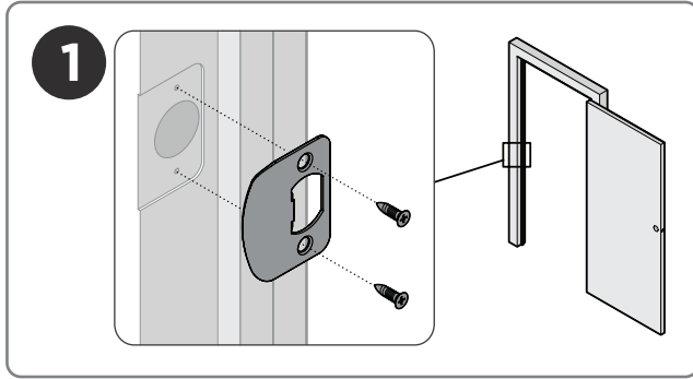
Install strike Instale la placa Instale la placa
